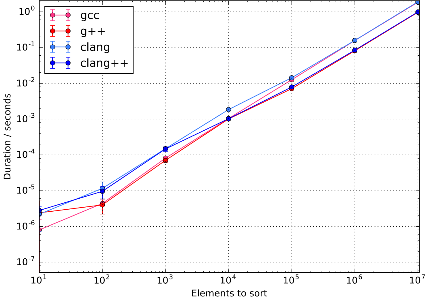
qsort vs. std::sort
