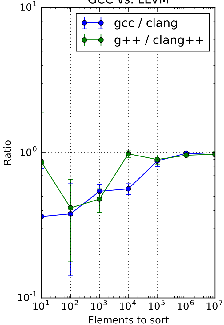
GCC vs. LLVM
