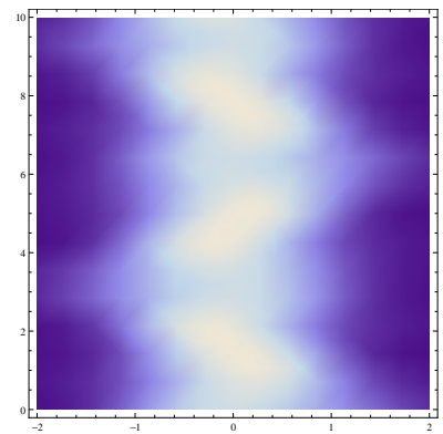
Abbildung 4: Dichte \rho_3
