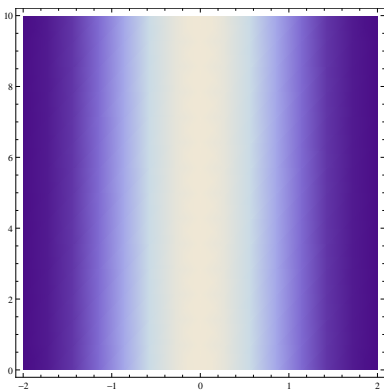
Abbildung 2: Dichte \rho_0
