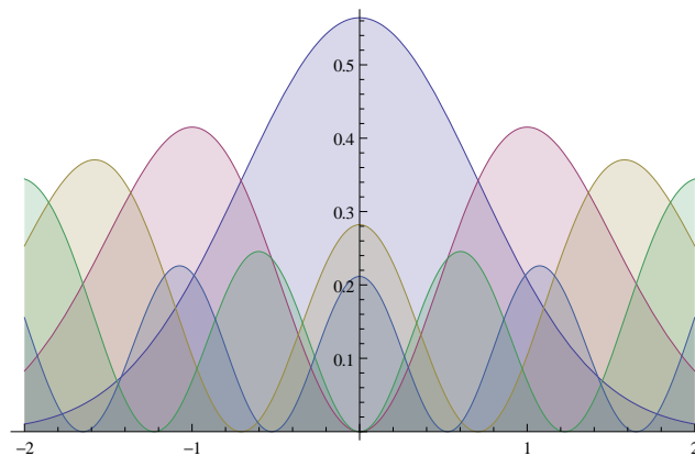
Abbildung 1: Plot von |\Psi_n(x, t)|^2 für n = 0, \dots, 3 . Horizontale Achse ist x , vertikale Achse ist die Wahrscheinlichkeitsdichte.
