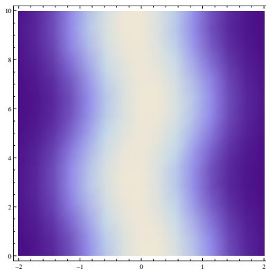
Abbildung 3: Dichte \rho_1
